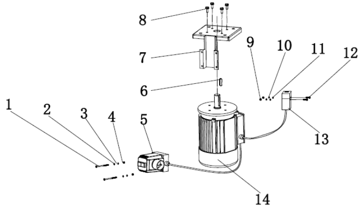
FIG.4 Motor
